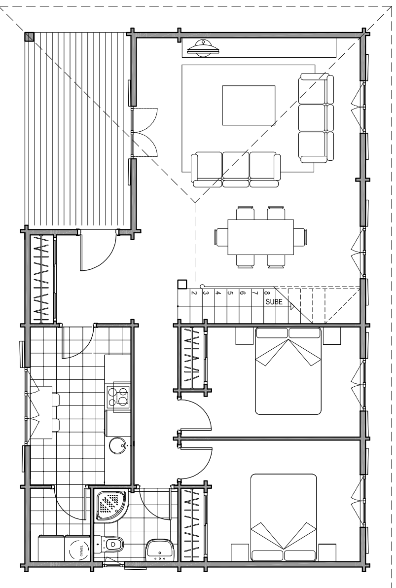
PLANTA BAJA
